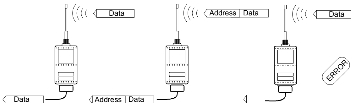
Рис. 5. Адресация приёма данных выключена (OFF-положение). Радиомодем передаёт все принятые пакеты данных по RS-интерфейсу
