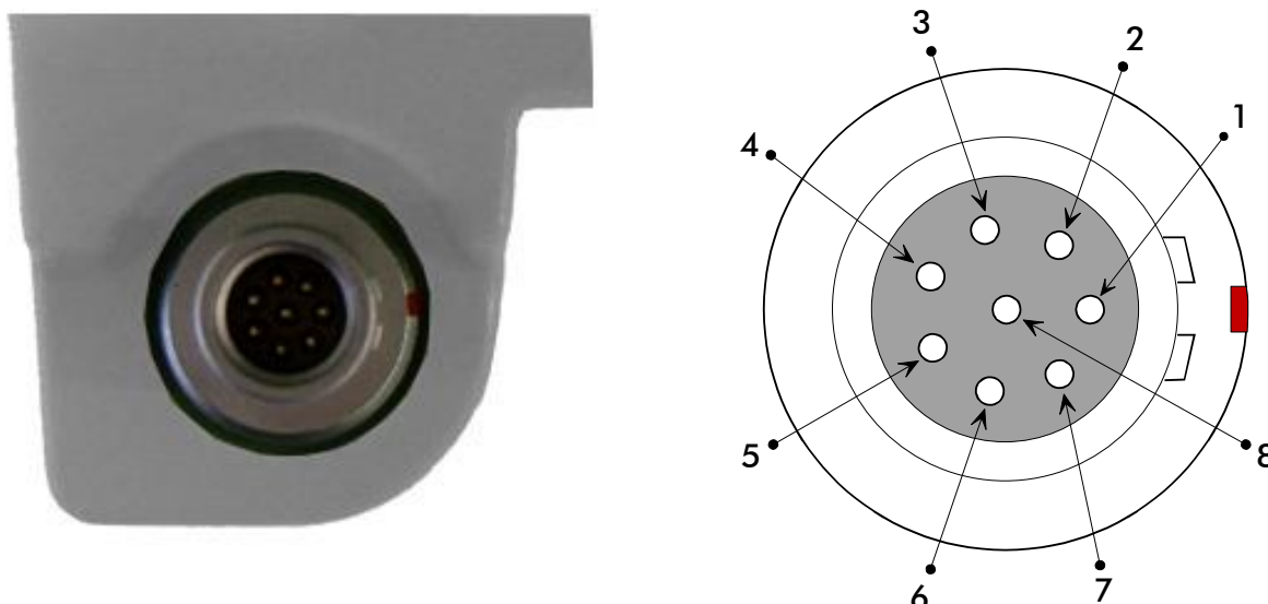
Рисунок 2.1 Разъем Lemo и расположение выводов
