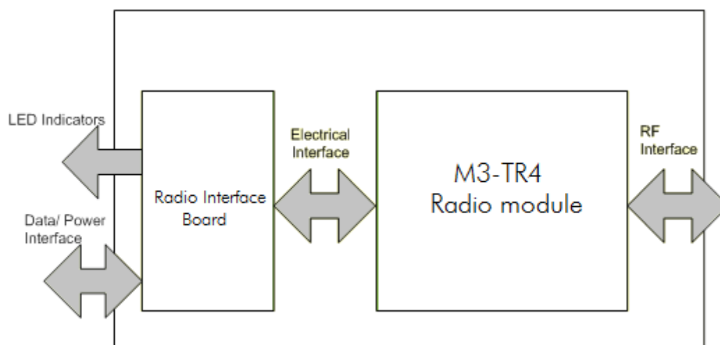
Рисунок 1.2 Блок-схема радиомодема для передачи данных GFU30
