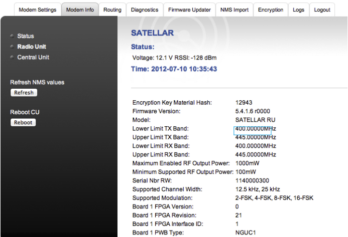
Рисунок 4.5: Информация о модеме / Страница настроек радиомодуля
