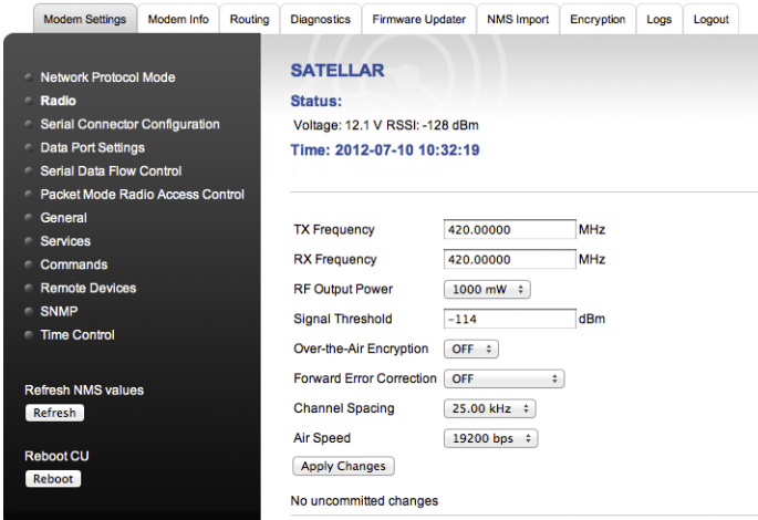
Рисунок 4.2: Страница настроек радио
